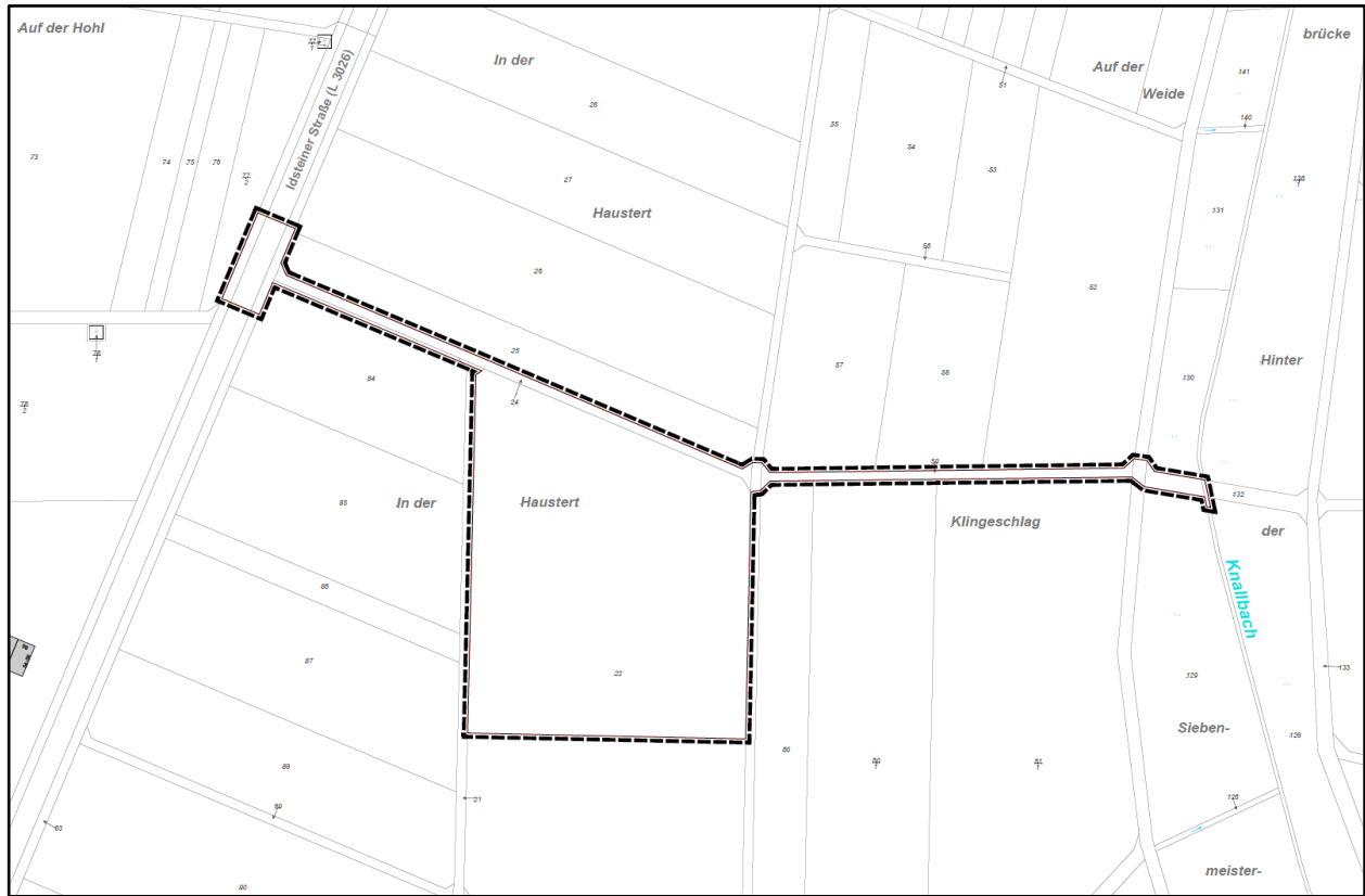
Abb. 1: Lage des räumlichen Geltungsbereichs des Bebauungsplanes „Sportanlage Walsdorf“; Idstein-Walsdorf (genordet, unmaßstäblich)
